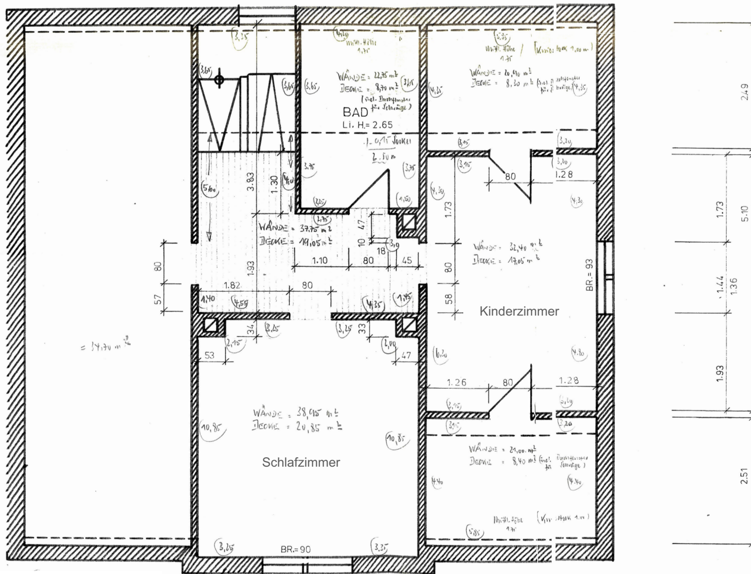
GRUNDRISS OBERGESCHOSS
